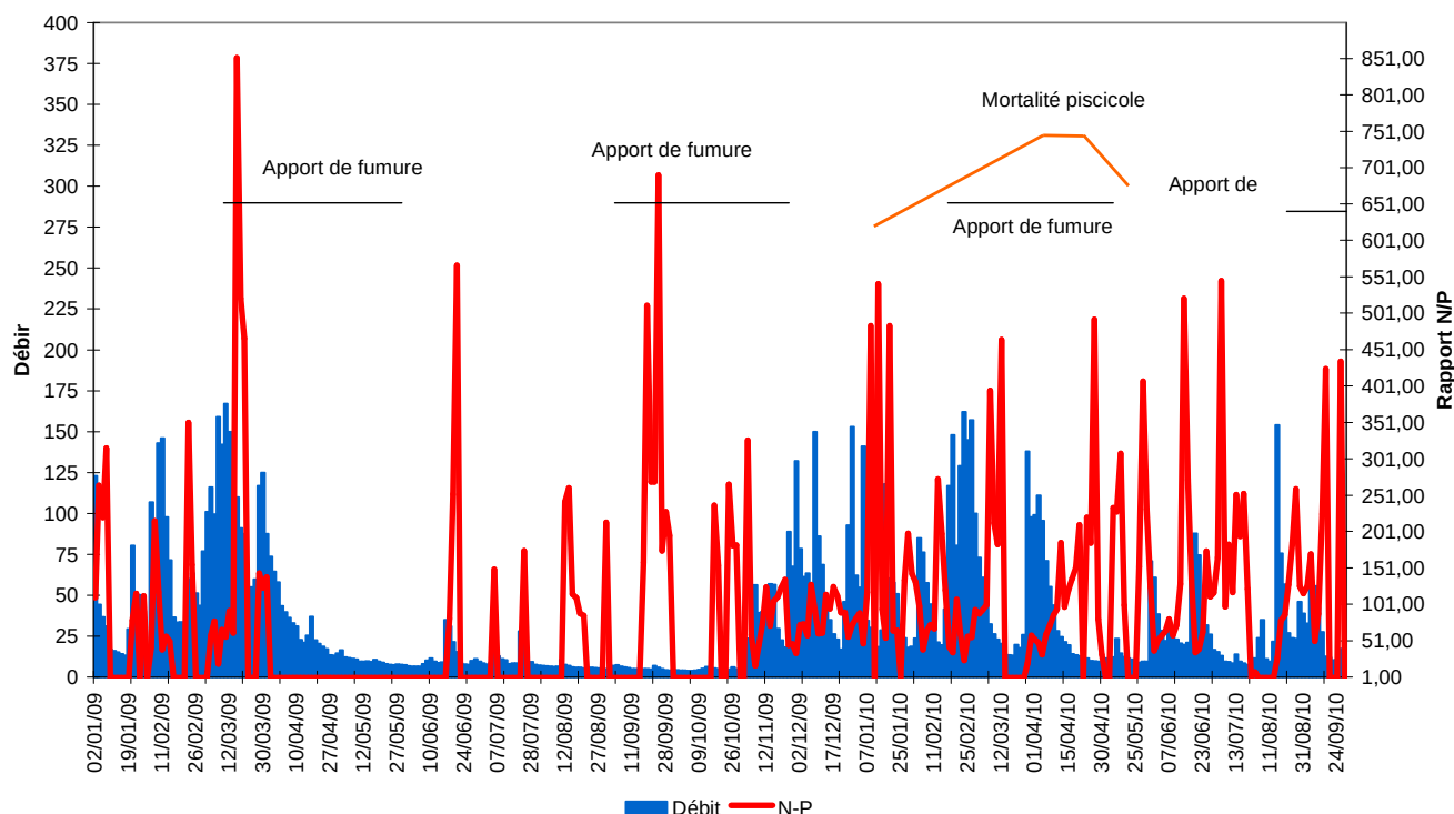
Figure 31: Evolution du rapport N/P à Chenecey de janvier 2009 à Octobre 2010.
