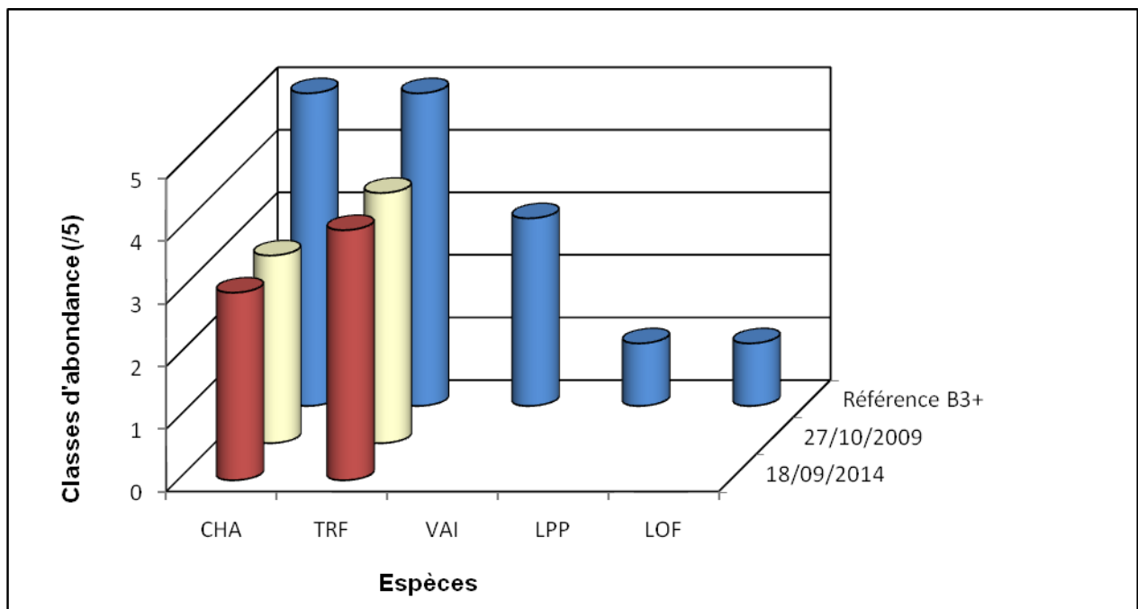
Figure 3.2. : Confrontation entre les peuplements observés et théoriques sur la station REVE 03
