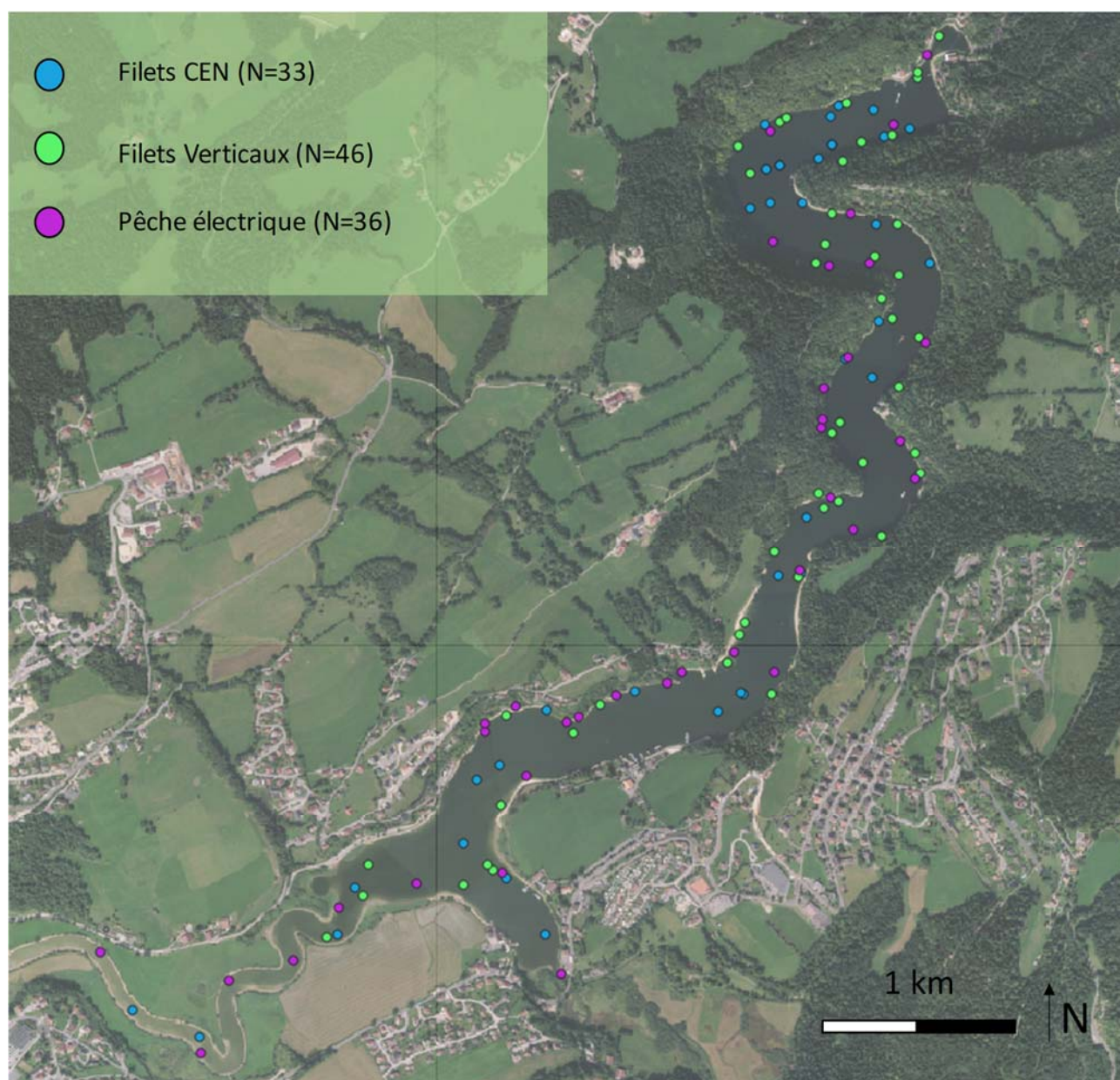
Figure 3.10 : Plan d'échantillonnage du lac de Chaillexon/Brenets.
