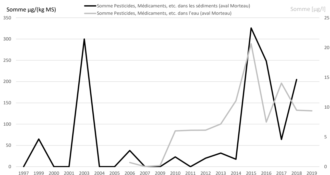
Figure 3.3 : Evolution de la teneur en micropolluants (pesticides, médicaments, produits de traitement, etc. ) dans les sédiments et les eaux de surface du Doubs en aval de Morteau (Données Agence de l'eau RMC).
