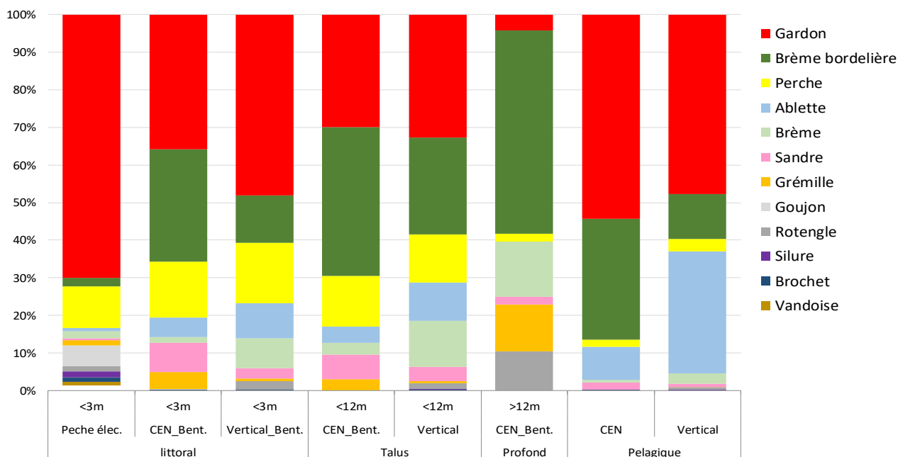
Figure 3.12 : Composition du peuplement de poissons capturé par compartiment du plan d'eau de Chaillexon/Brenets.
