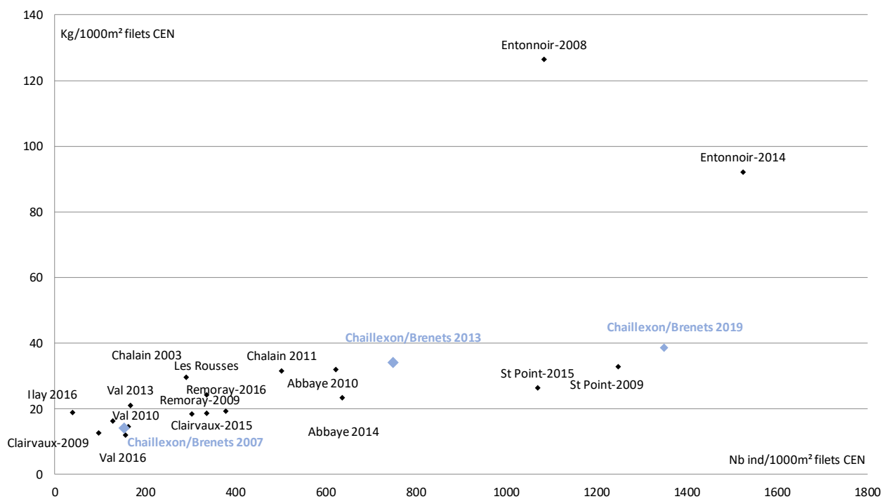
Figure 3.29 : Rendement de pêche comparé aux filets CEN des lacs naturels régionaux morphologiquement et typologiquement proches (Données OFB).
