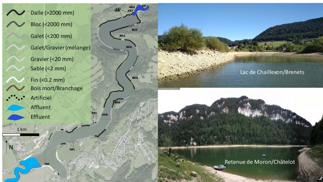
Figure 3.7 : Carte des habitats littoraux du lac de Chaillexon/Brenets et photographies d'illustration.
