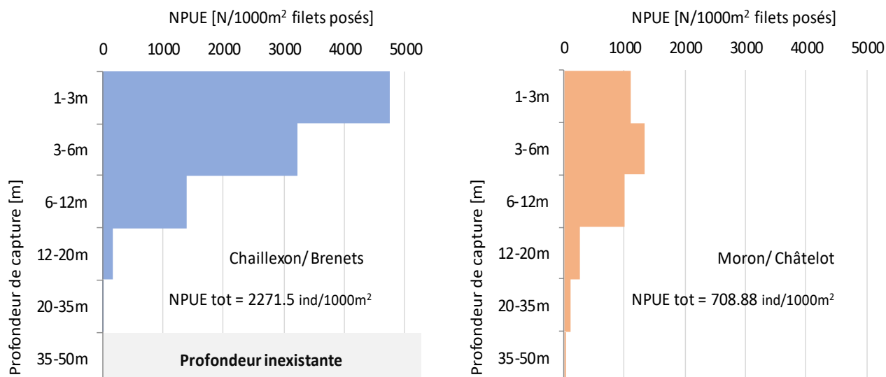
Figure 3.17 : Répartition verticale des captures réalisés sur le fond du lac à l'aide des filets benthiques CEN.
