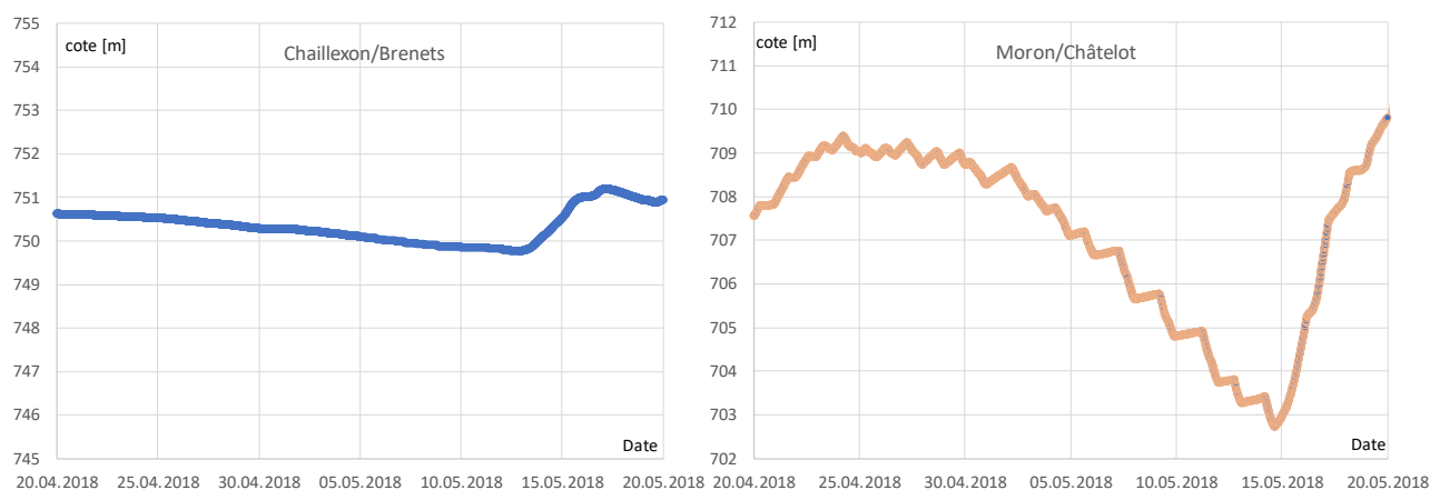
Figure 4.3 : Exemple de l'évolution des niveaux d'eau comparée d'un plan d'eau à l'autre en début de période de reproduction des cyprinidés (données OFEV et Groupe E).
