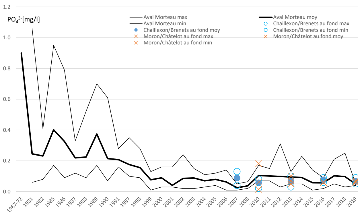
Figure 3.1 : Evolution de la teneur en orthophosphates des eaux de surface (Données Agence de l'eau RMC).
