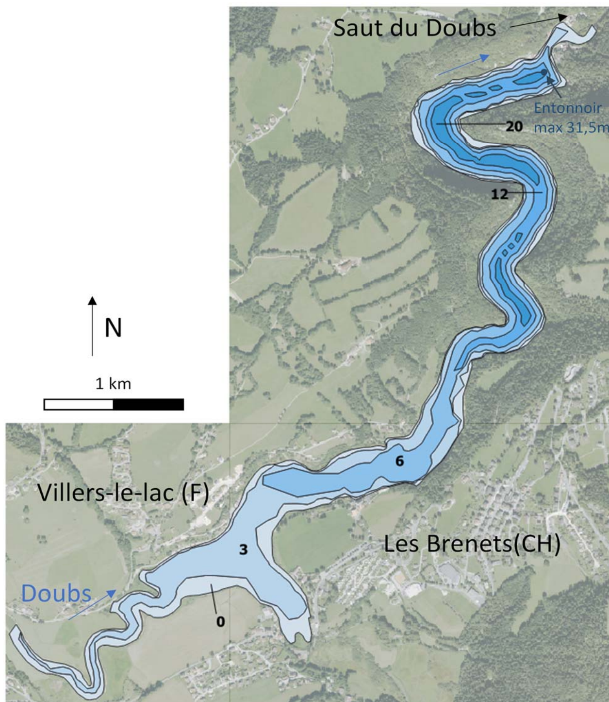
Figure 1.1 : Bathymétrie du lac de Chaillexon/Brenets (Données OFB)
