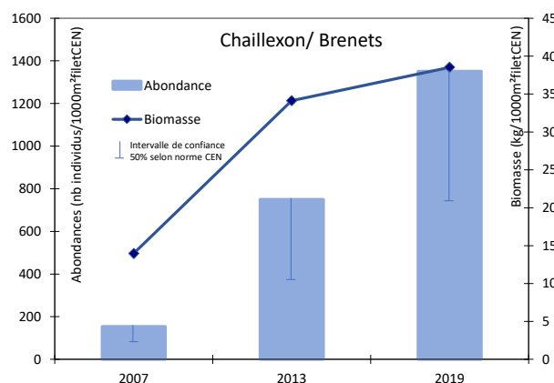
Figure 3.27 : Evolution des rendements de pêche aux filets benthiques CEN de 2007 à 2019 sur Chaillexon/Brenets et Moron/Châtelot (données OFB)
