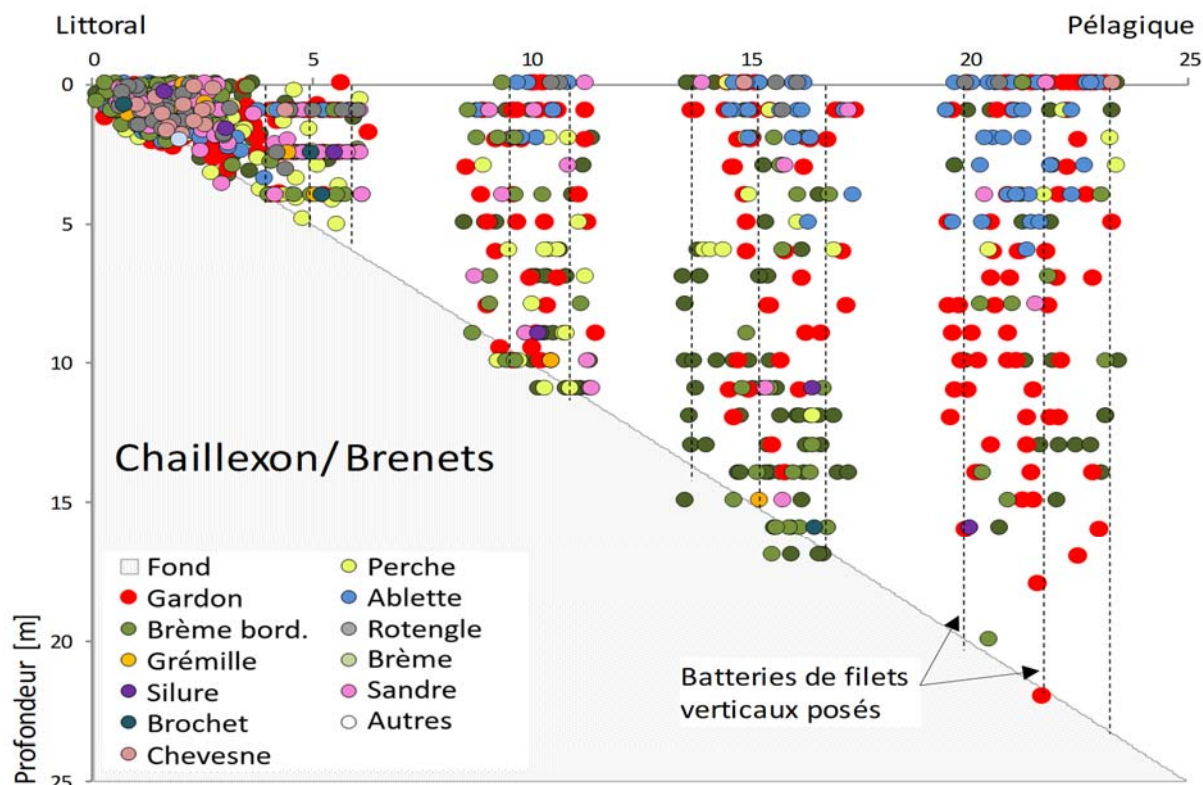
Figure 3.14 : Répartition spatiale des captures réalisées à partir des filets verticaux sur le lac de Chaillexon/Brenets
